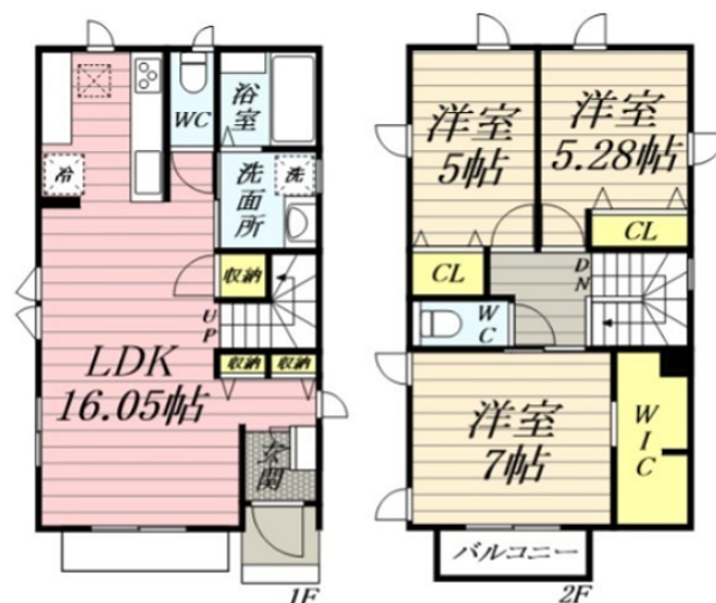
【間取り図】
