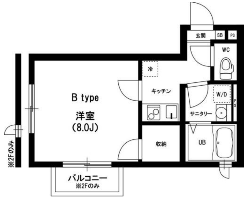
【間取り図】
