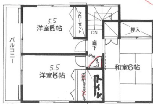
【2階平面図】
