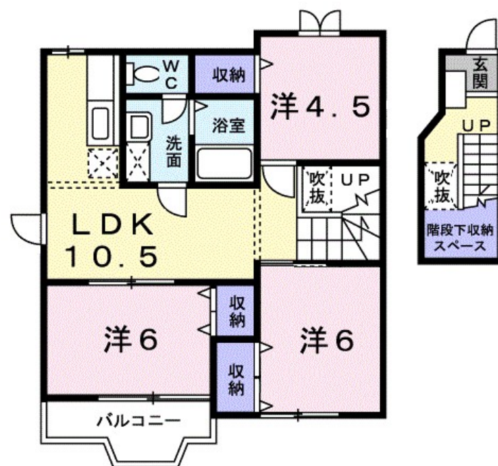
【間取り図】
