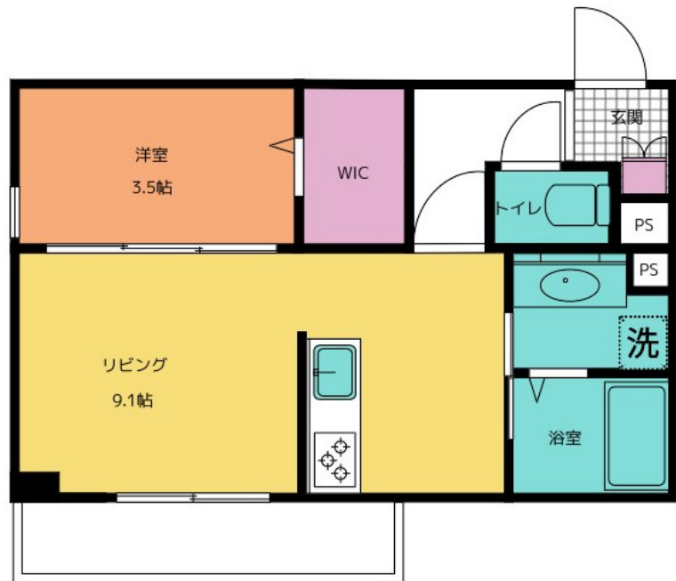
【間取り図】
