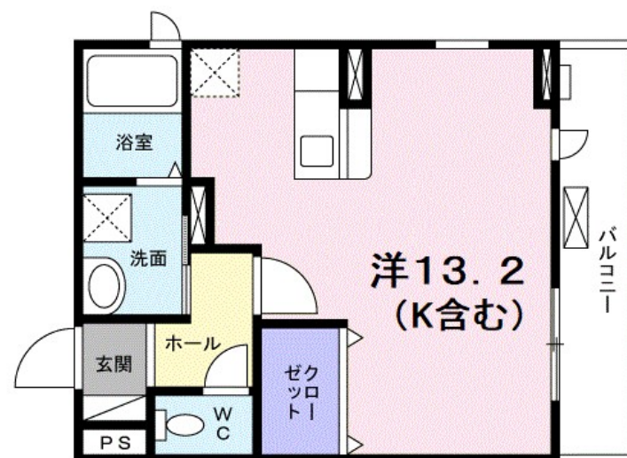
【間取り図】
