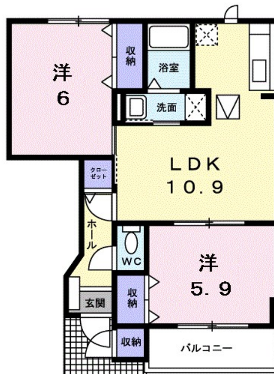
【間取り図】
