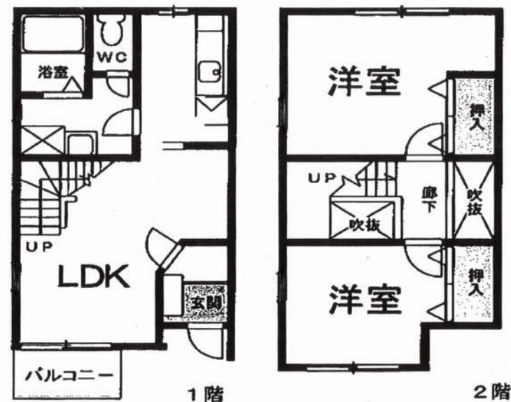
【間取り図】
