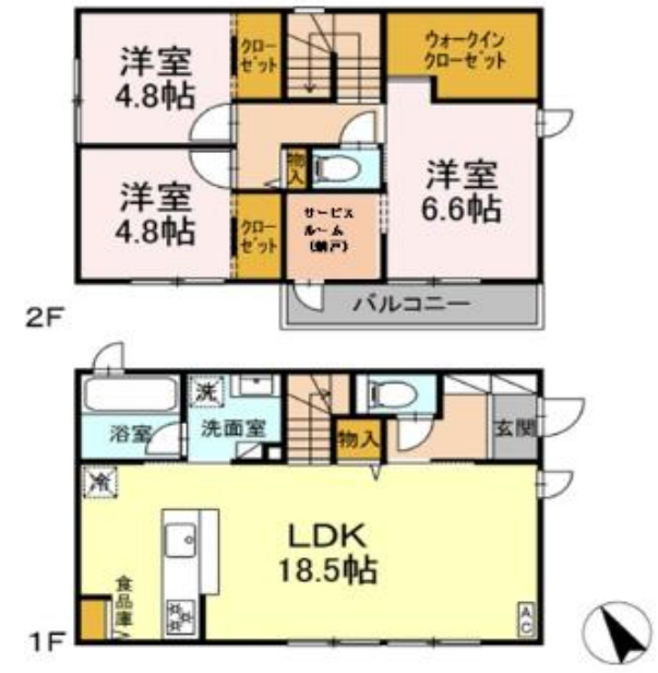
【間取り図】
