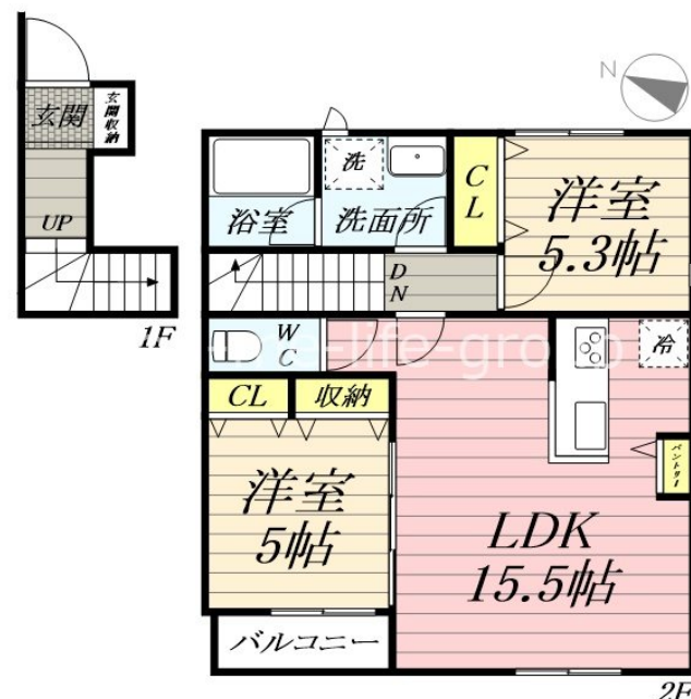
【間取り図】
